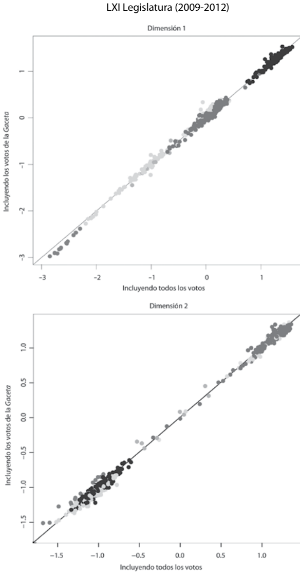
GRÁFICA 3B. Comparación coordinada por coordinada de los puntos ideales estimados con todos los votos (eje x ) y con los votos publicados en la Gaceta (eje y )
